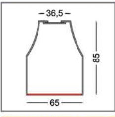
117500 | Sıva üstü profil
