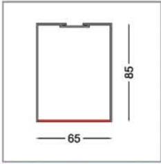
101500 | Sıva üstü profil
