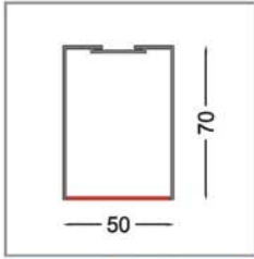
106500 | Sıva üstü profil
