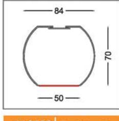
112500 | Sıva üstü profil
