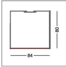
163500 | Sıva üstü profil
