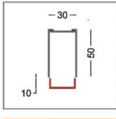
110500 | Sıva üstü profil
