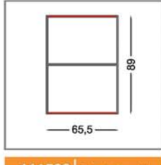
111500 | Sıva üstü profil
