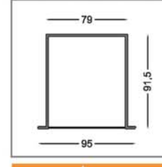
161500 | Sıva altı profil
