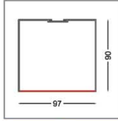
109500 | Sıva üstü profil
