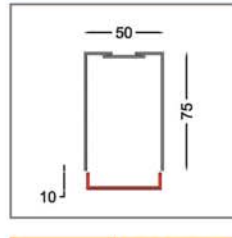
116500 | Sıva üstü profil
