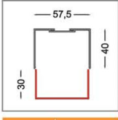
103500 | Sıva üstü profil
