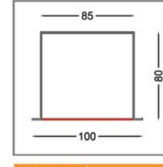
119500 | Sıva altı profil
