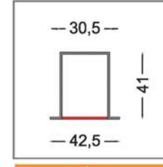
160500 | Sıva altı profil
