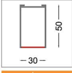
114500 | Sıva üstü profil
